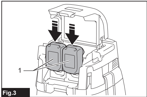
Fig.3 ► 1. Batterie
